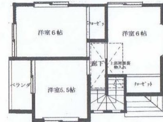
2階平面図
